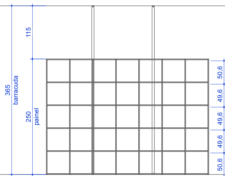
ELEVAÇÃO - PAINEL 7A escala 1:50
