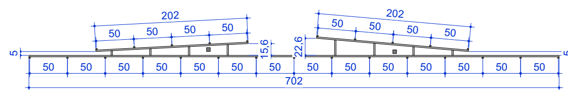
PLANTA - PAINEL 6 escala 1:50
