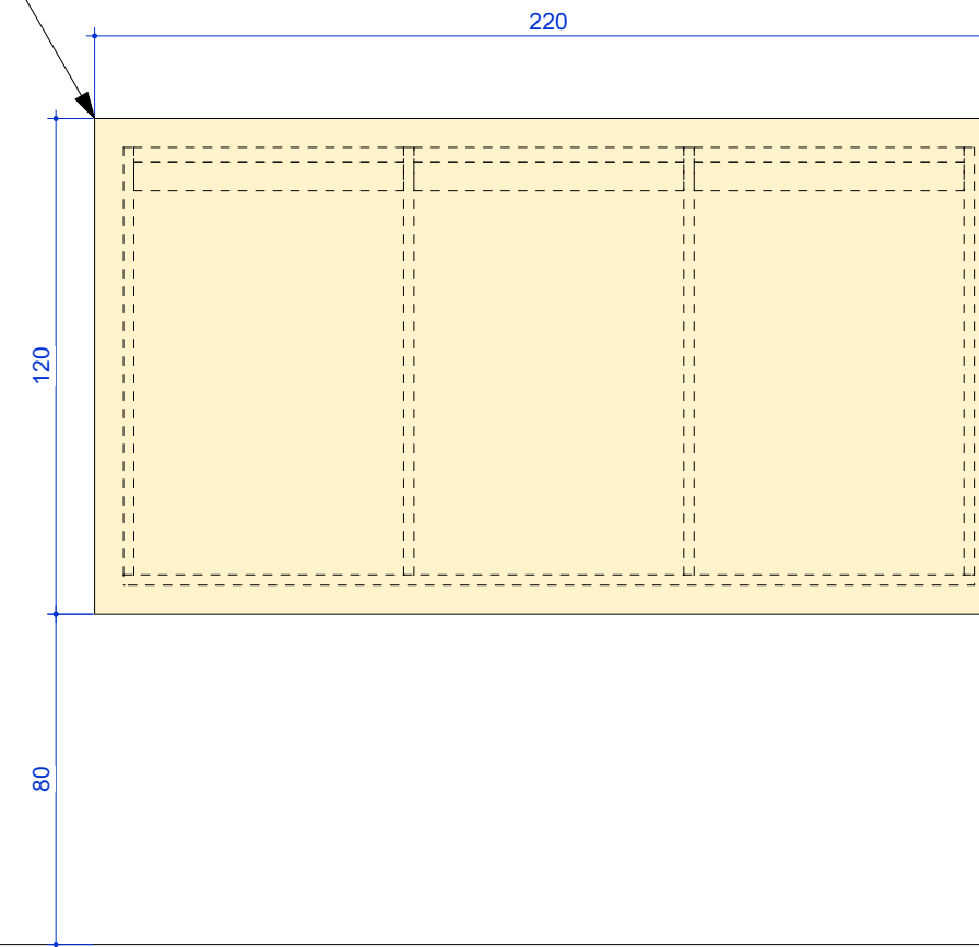
PLANTA - PAINEL QATAR escala 1:20
