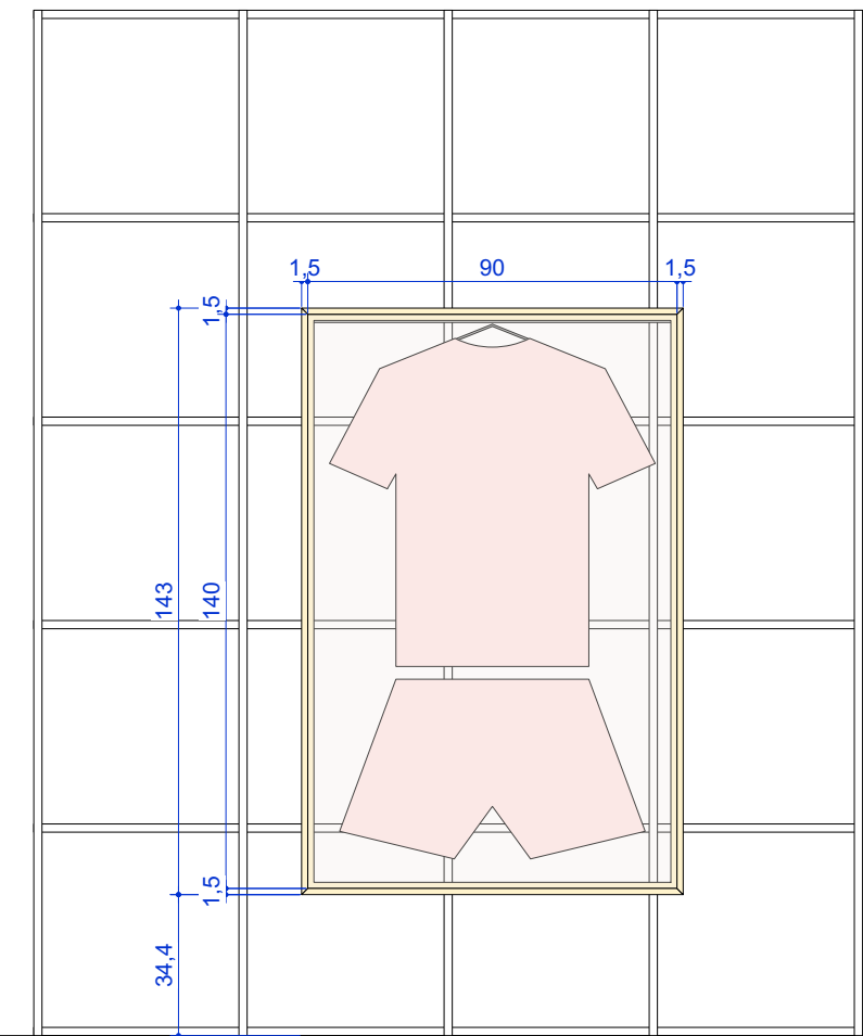
ELEVAÇÃO FRONTAL - CAIXA DE ACRÍLICO escala 1:20
