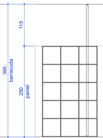
ELEVAÇÃO - PAINEL 2 B1 escala 1:50
