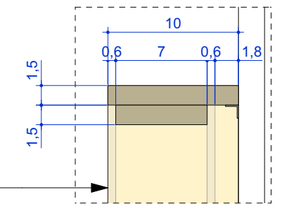
DETALHE 02 - CAIXA DE ACRÍLICO escala 1:20
