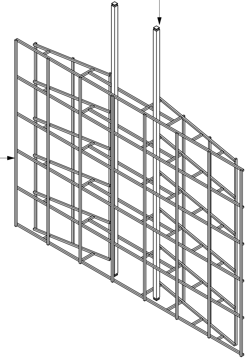
EXEMPLO CONSTRUTIVO ISOMETRICA - ESTRUTURA PAINEL escala 1:20
