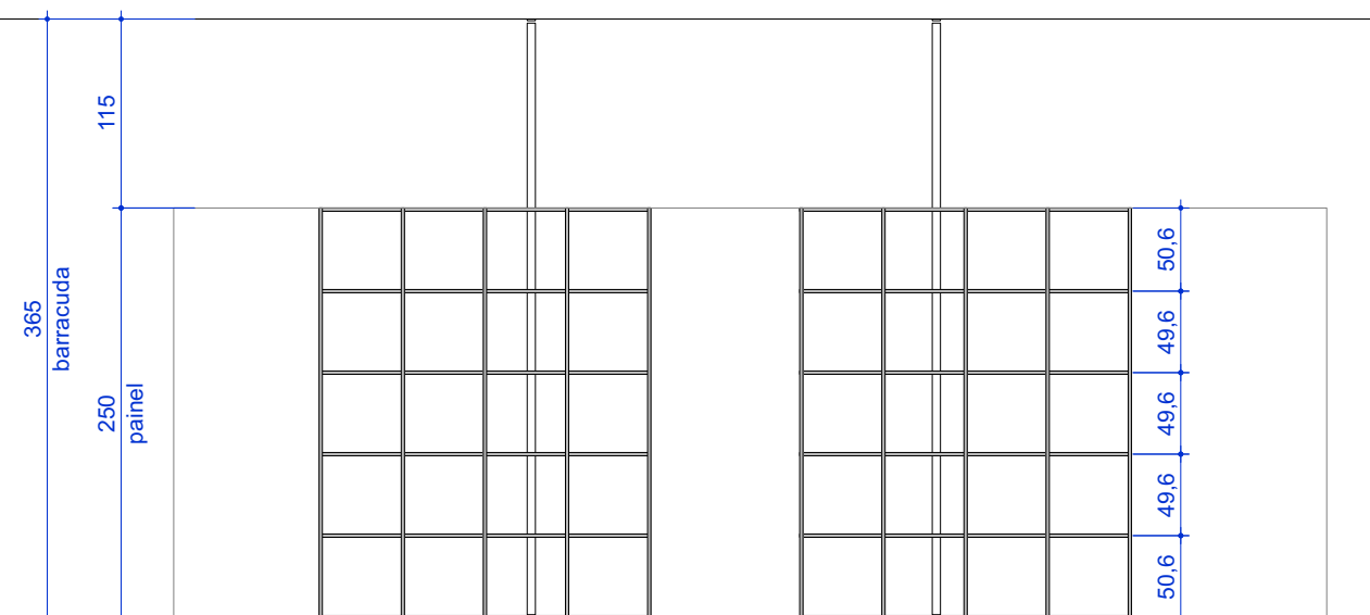
ELEVAÇÃO - PAINEL 6B1 escala 1:50
