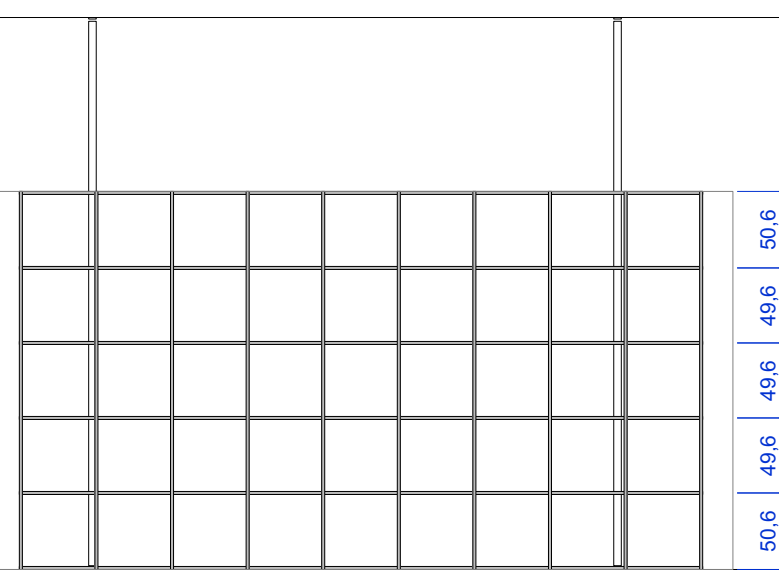
ELEVAÇÃO - PAINEL 3B2 escala 1:50
