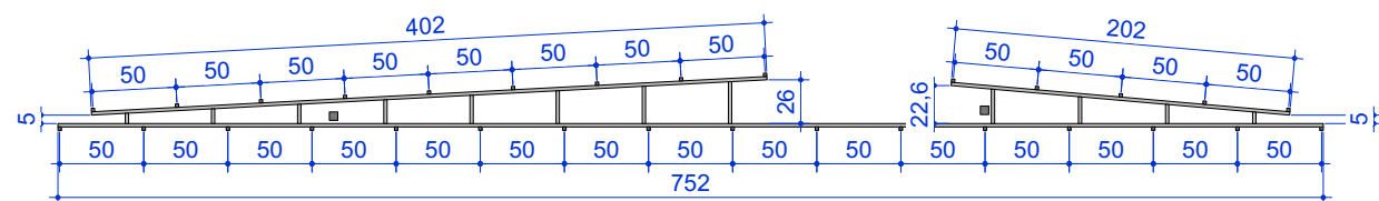
PLANTA - PAINEL 5 escala 1:50
