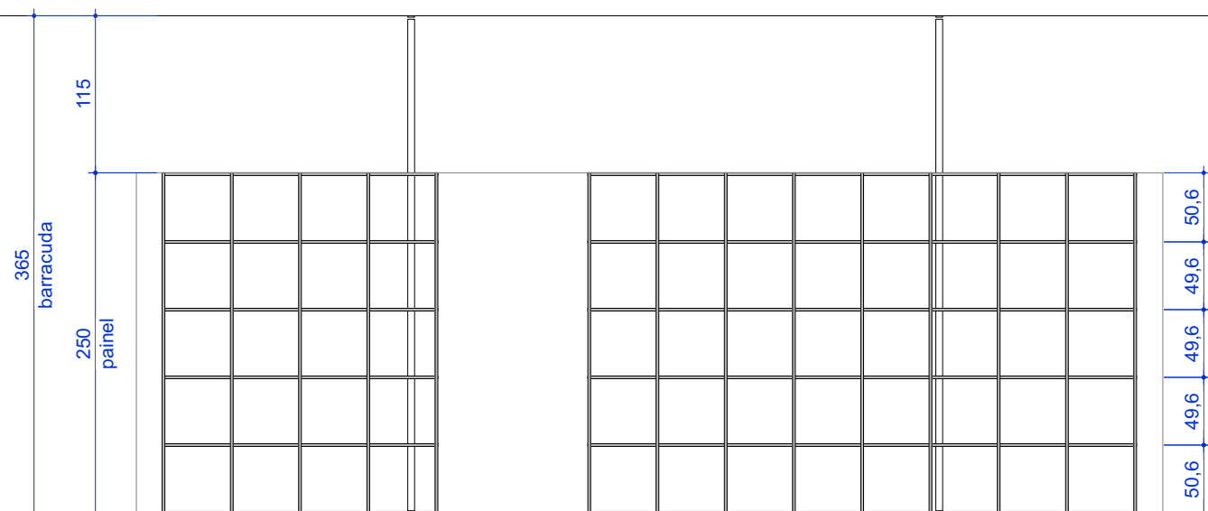
ELEVAÇÃO - PAINEL 5B1 escala 1:50
