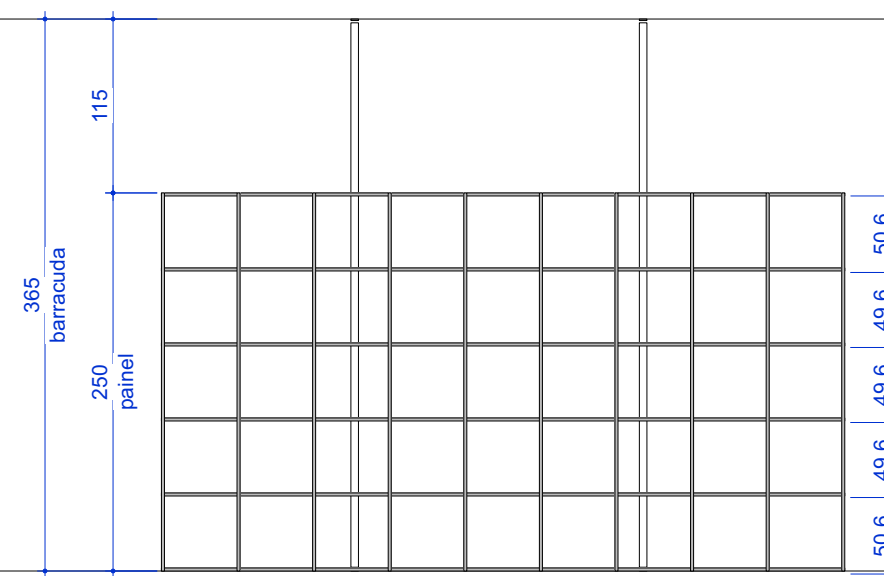
ELEVAÇÃO - PAINEL 9A escala 1:50
