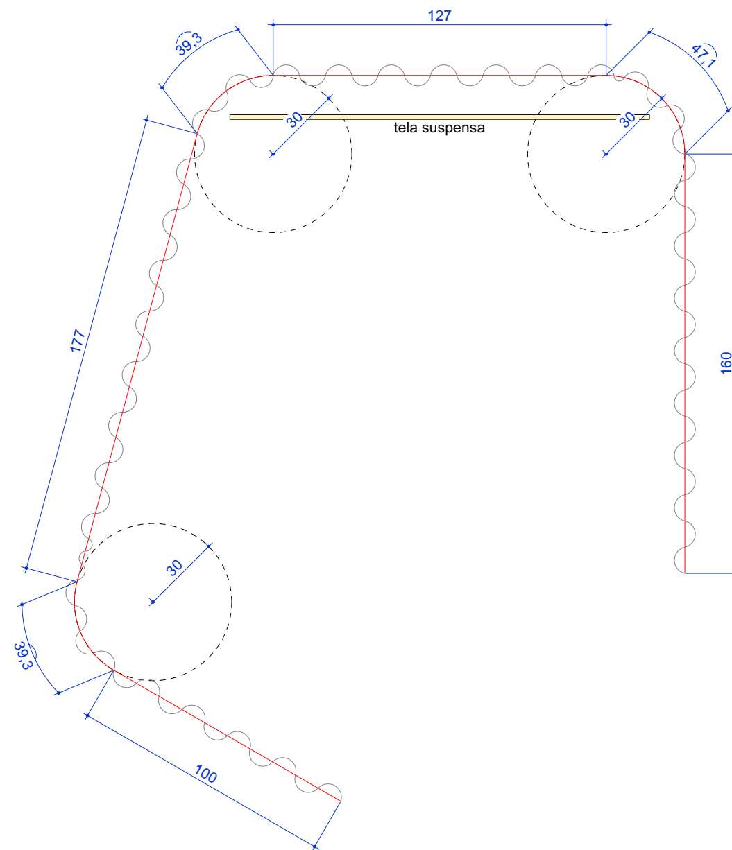
2x UNIDADES PLANTA - SALAS DE VÍDEO 1 e 2 escala 1:20
