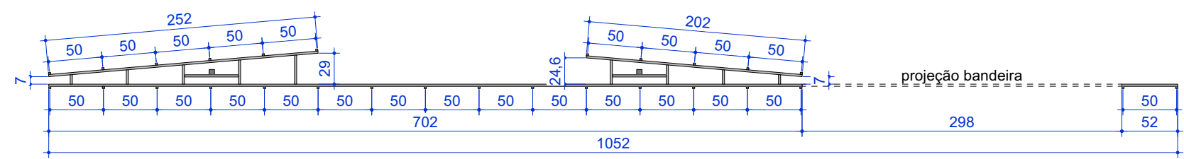
PLANTA - PAINEL 1 escala 1:50
