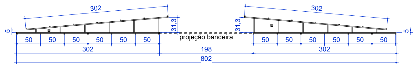
PLANTA - PAINEL 4 escala 1:50
