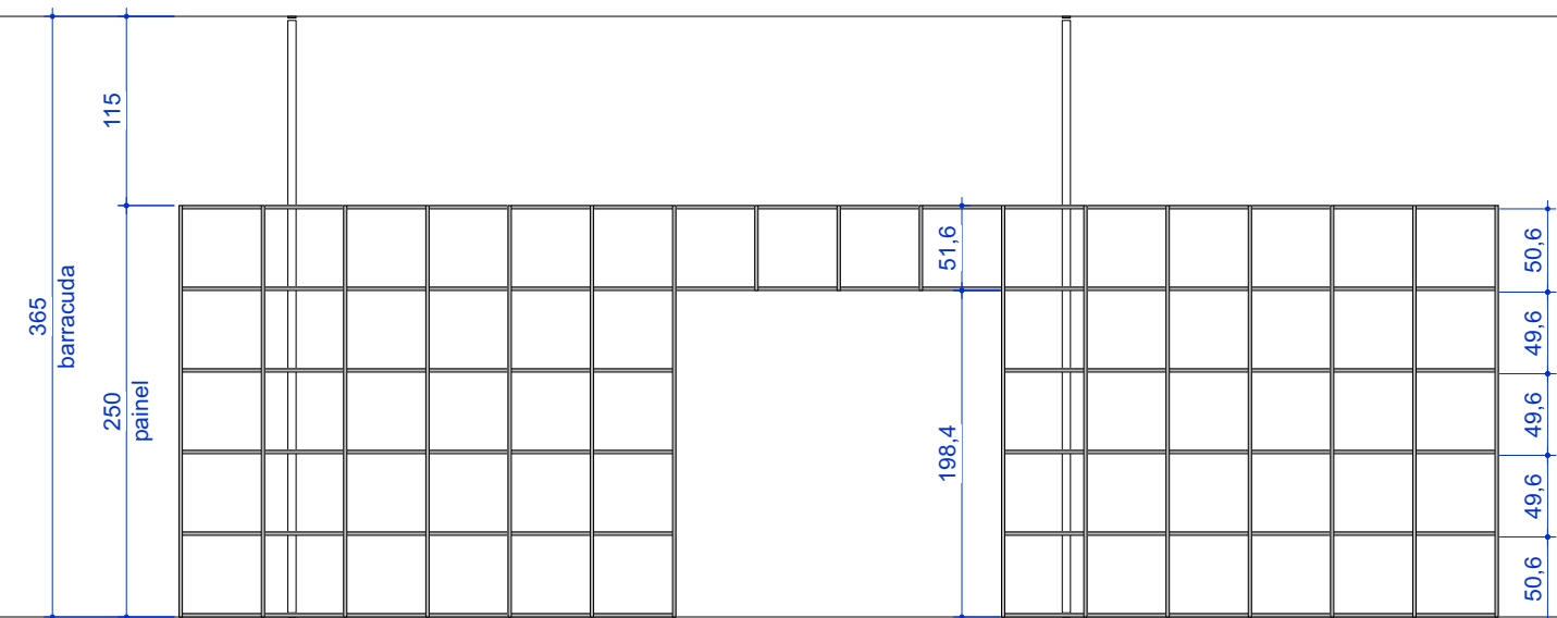
ELEVAÇÃO - PAINEL 4A escala 1:50
