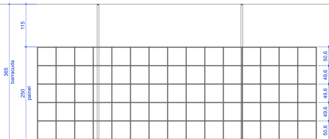
ELEVAÇÃO - PAINEL 5A escala 1:50
