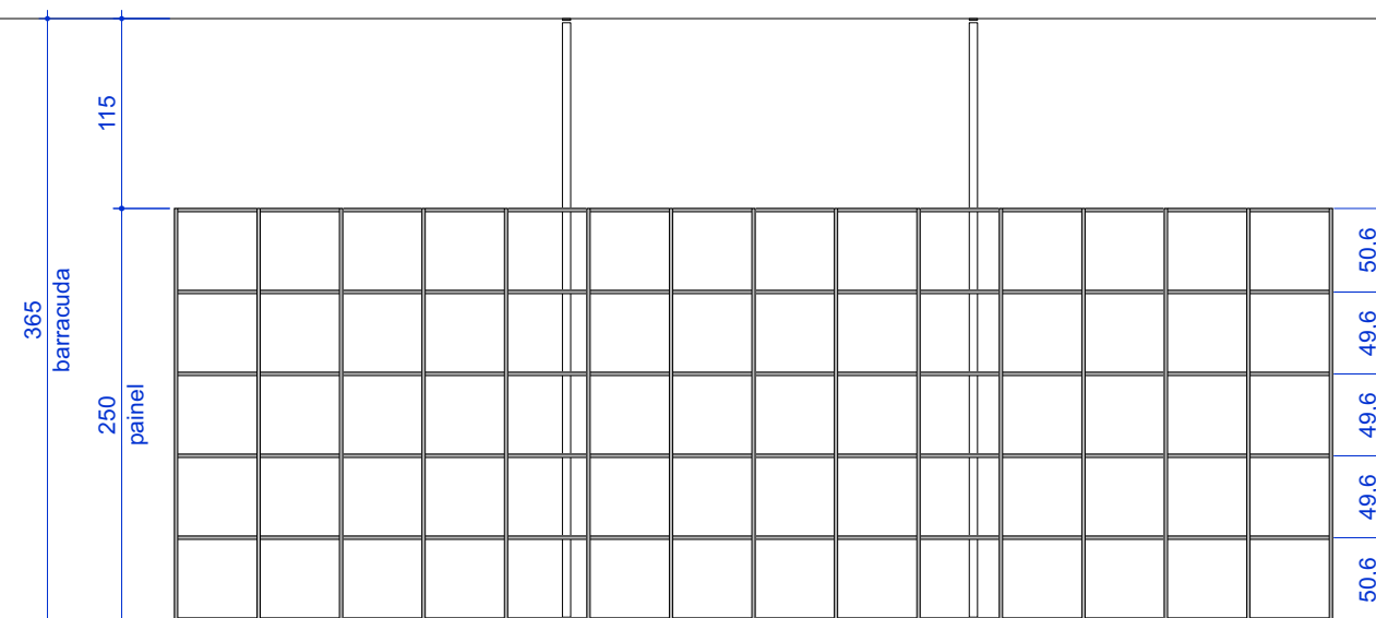
ELEVAÇÃO - PAINEL 6A escala 1:50
