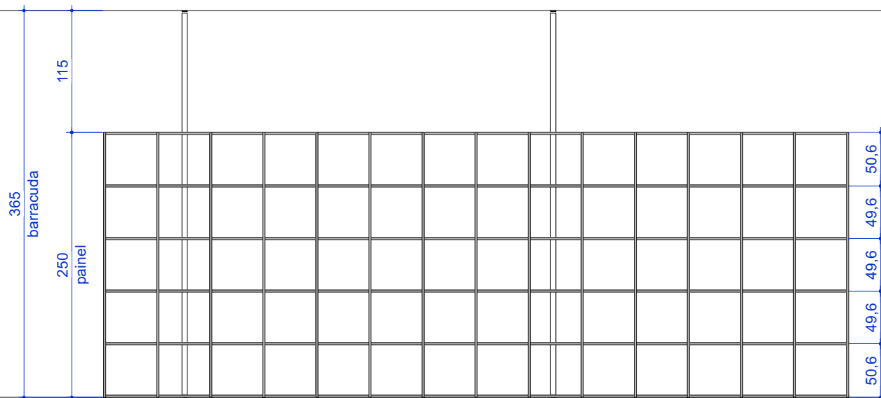
ELEVAÇÃO - PAINEL 3A escala 1:50
