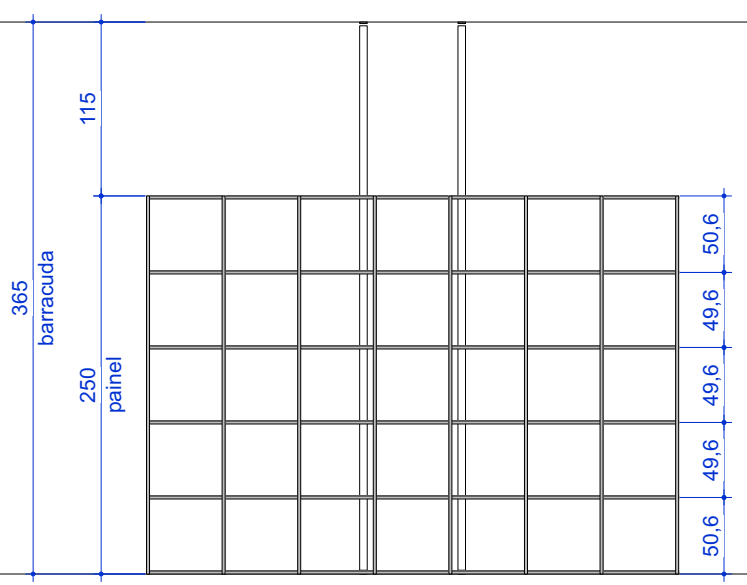
ELEVAÇÃO - PAINEL 2A escala 1:50
