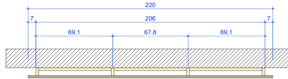
PLANTA - PAINEL QATAR escala 1:20
