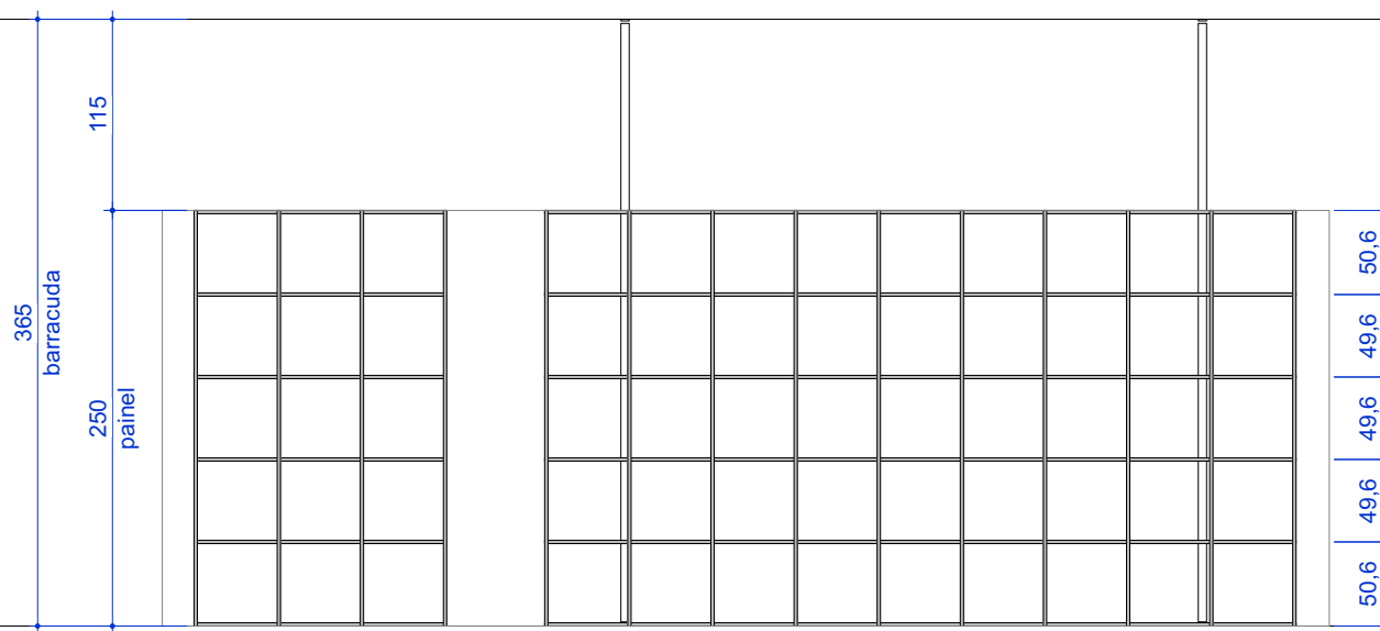
ELEVAÇÃO - PAINEL 3B1 escala 1:50
