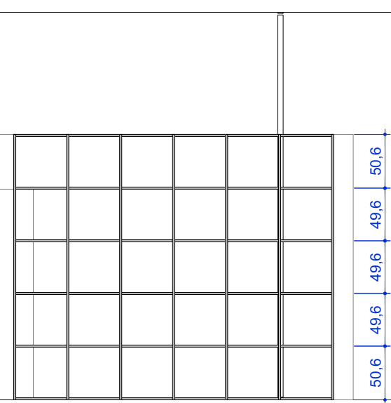
ELEVAÇÃO - PAINEL 4B2 escala 1:50
