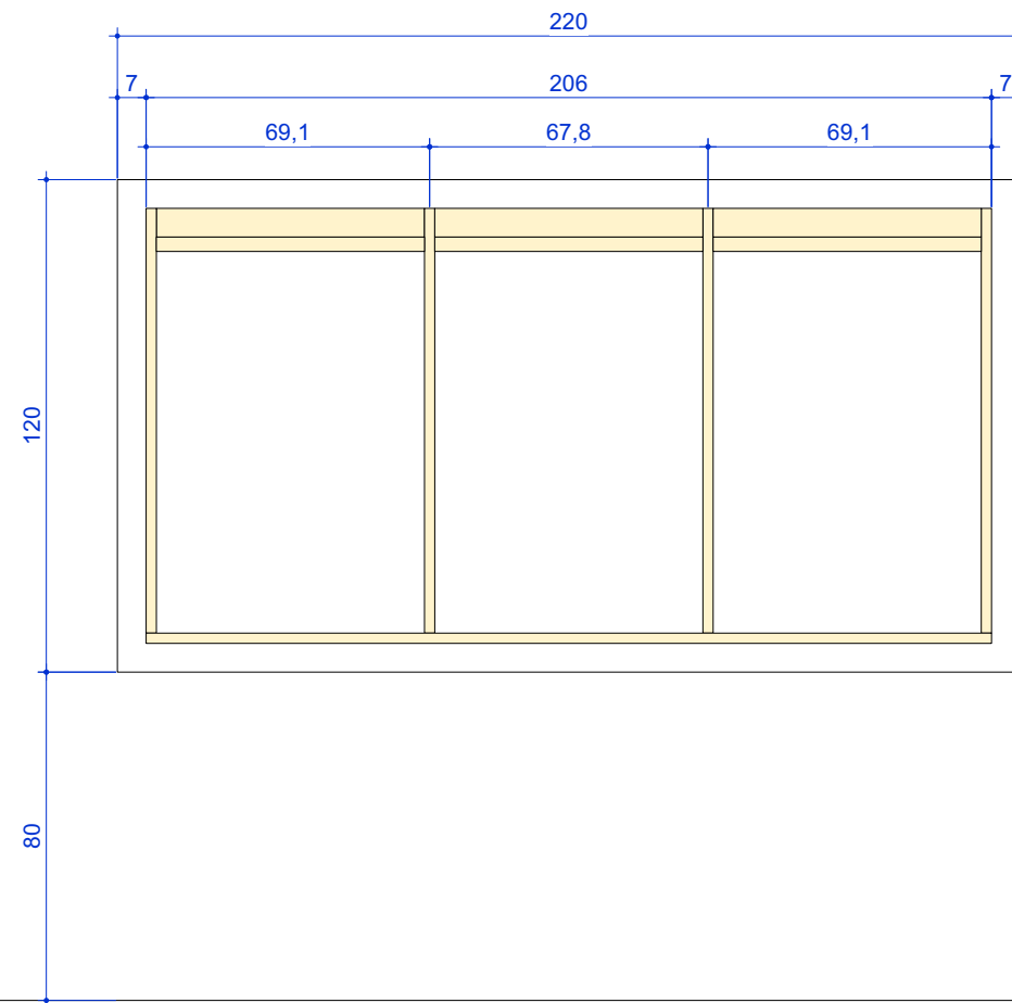
ELEVAÇÃO POSTERIOR - PAINEL QATAR escala 1:20
