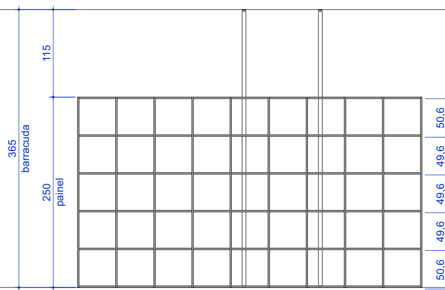
ELEVAÇÃO - PAINEL 8A escala 1:50
