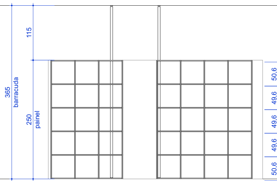
ELEVAÇÃO - PAINEL 8B1 escala 1:50
