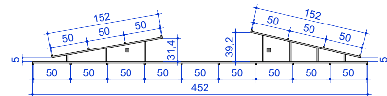
PLANTA - PAINEL 9 escala 1:50
