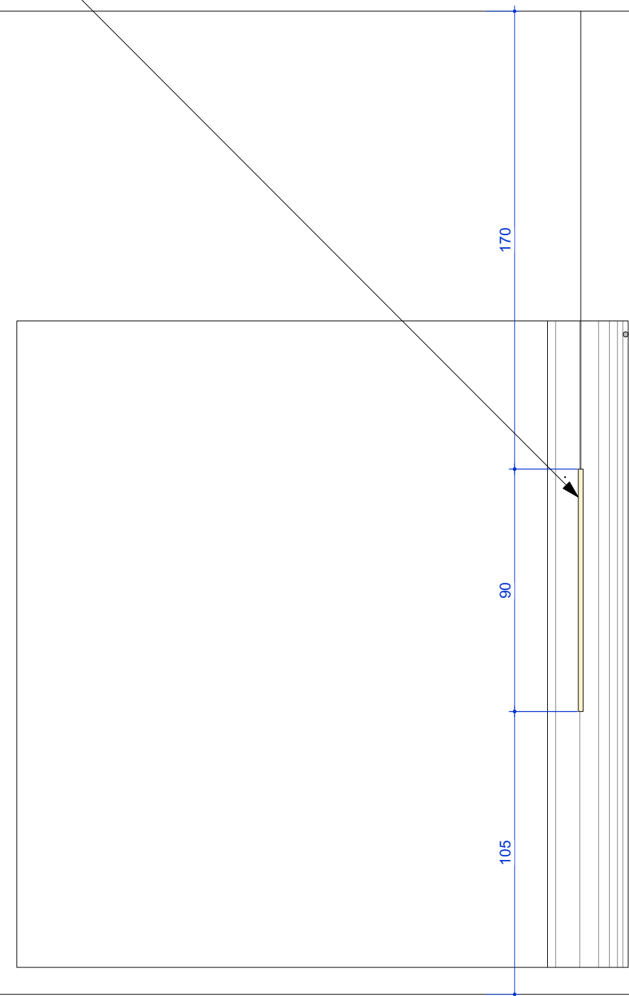
CORTE - TELA PARA PROJEÇÃO escala 1:20
