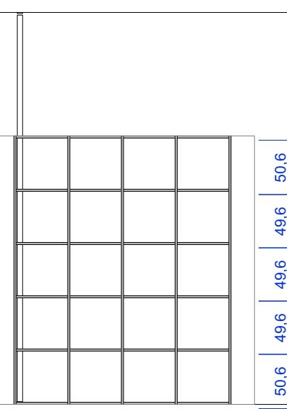
ELEVAÇÃO - PAINEL 8B2 escala 1:50
