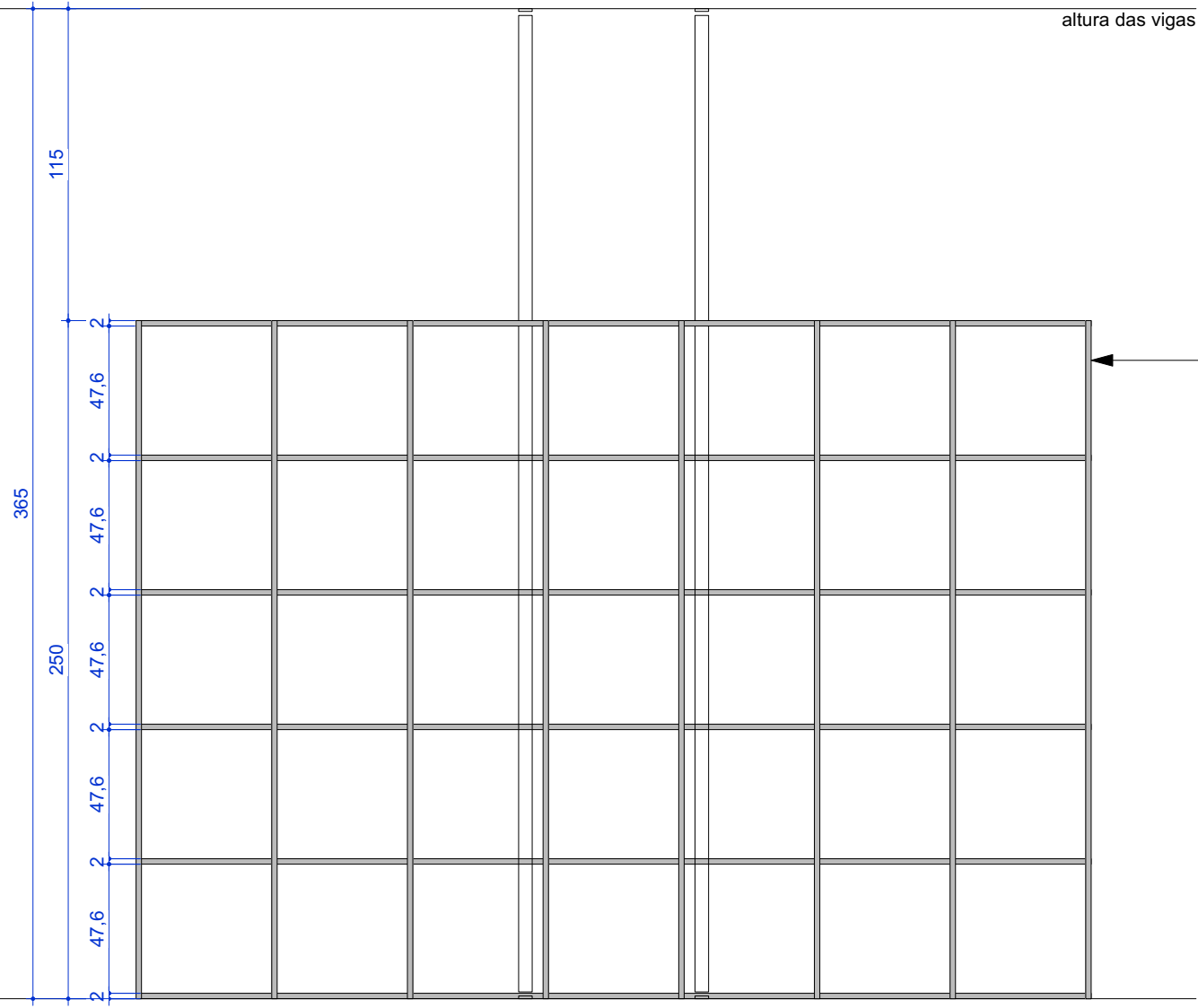
EXEMPLO CONSTRUTIVO ELEVAÇÃO - ESTRUTURA PAINEL escala 1:20
