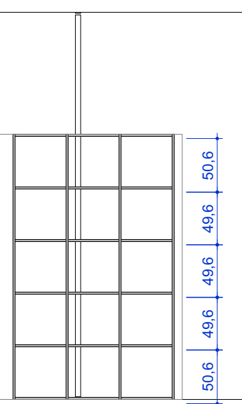
ELEVAÇÃO - PAINEL 7B2 escala 1:50
