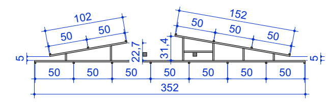
PLANTA - PAINEL 2 escala 1:50
