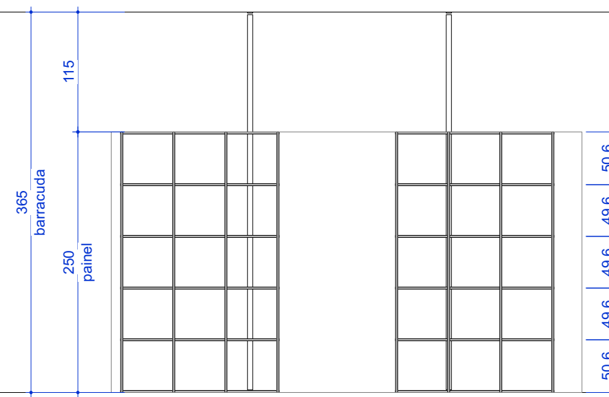
ELEVAÇÃO - PAINEL 9B1 escala 1:50
