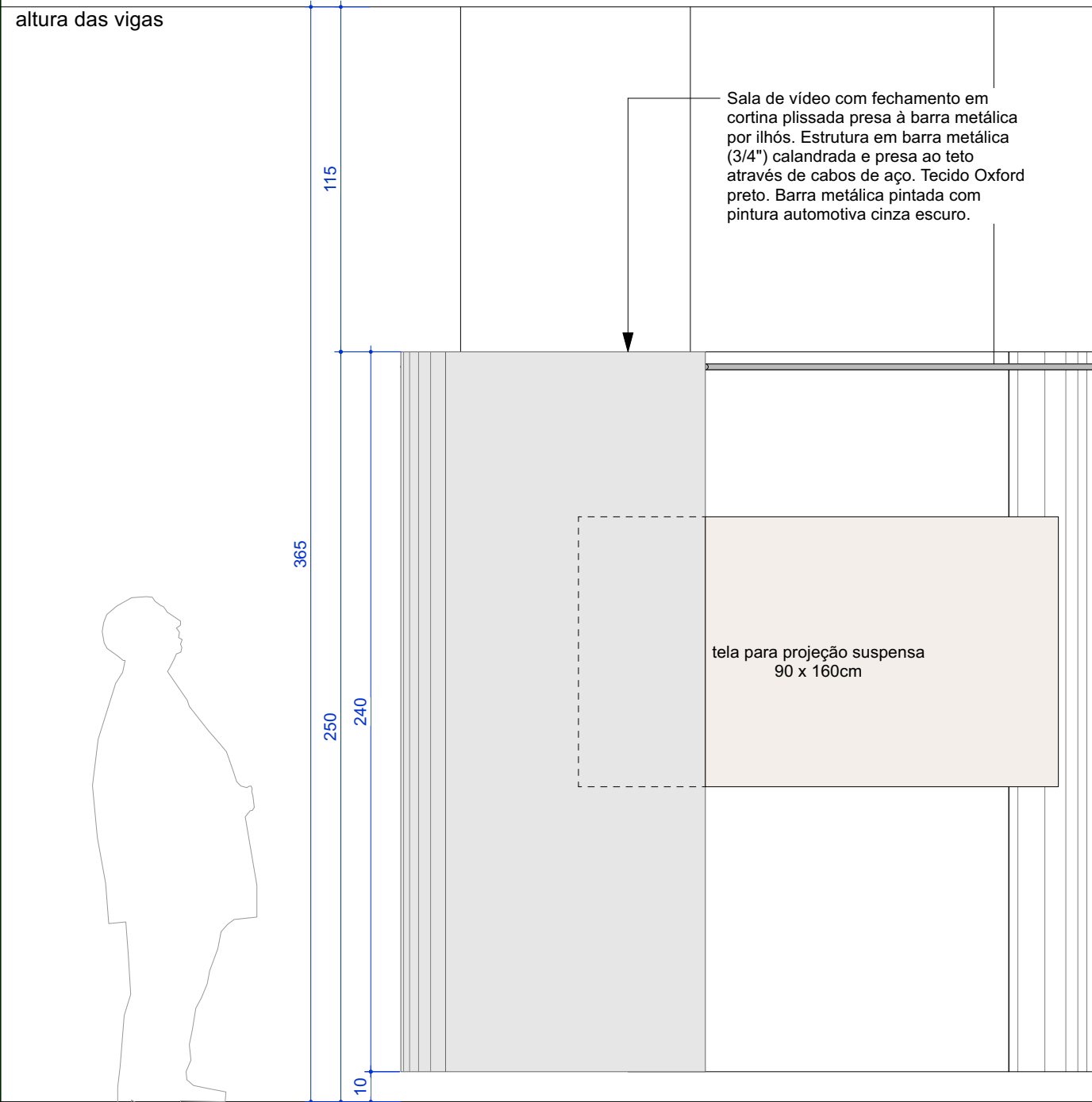
ELEVAÇÃO ESQUEMÁTICA - SALAS DE VÍDEO escala 1:20
