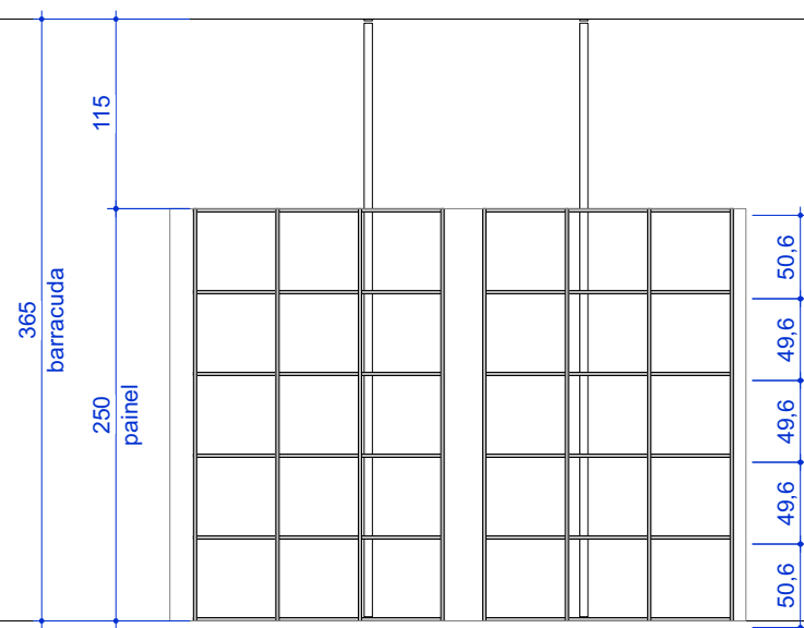
ELEVAÇÃO - PAINEL 7B1 escala 1:50
