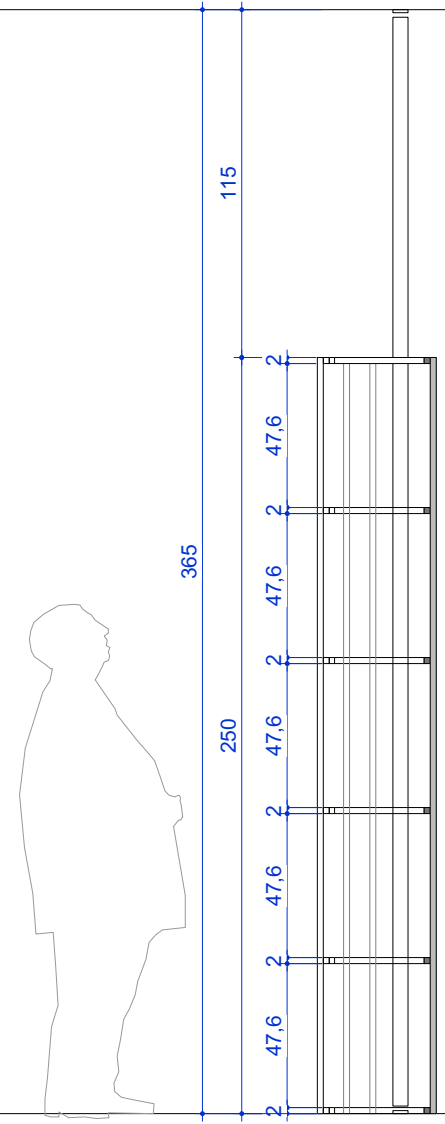
EXEMPLO CONSTRUTIVO CORTE - ESTRUTURA PAINEL escala 1:20
