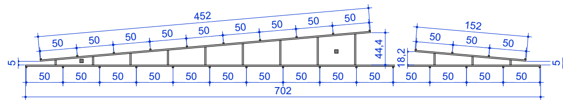
PLANTA - PAINEL 3 escala 1:50
