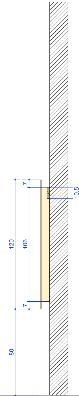
CORTE - PAINEL QATAR escala 1:20
