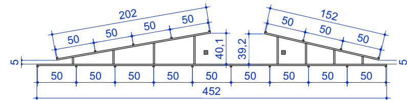
PLANTA - PAINEL 8 escala 1:50
