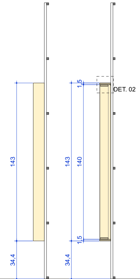
CORTES - CAIXA DE ACRÍLICO escala 1:20
