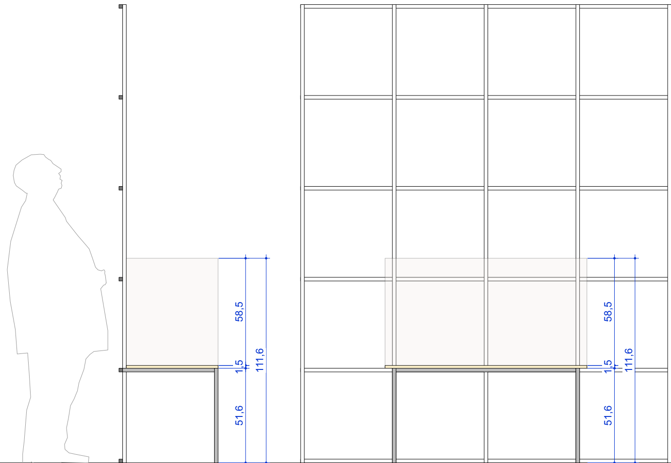
ELEVAÇÃO FRONTAL - BASE COM CÚPULA DE ACRÍLICO escala 1:20
