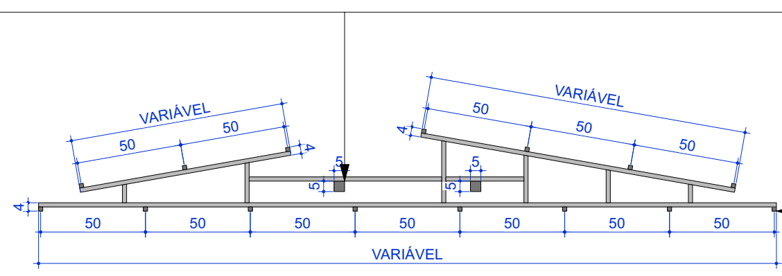
EXEMPLO CONSTRUTIVO PLANTA - ESTRUTURA PAINEL escala 1:20
