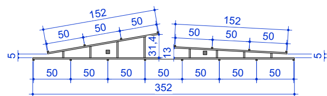
PLANTA - PAINEL 7 escala 1:50
