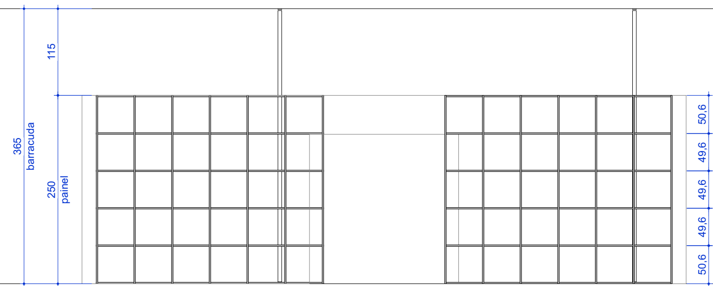
ELEVAÇÃO - PAINEL 4B1 escala 1:50
