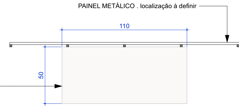
PLANTA - BASE COM CÚPULA DE ACRÍLICO escala 1:20
