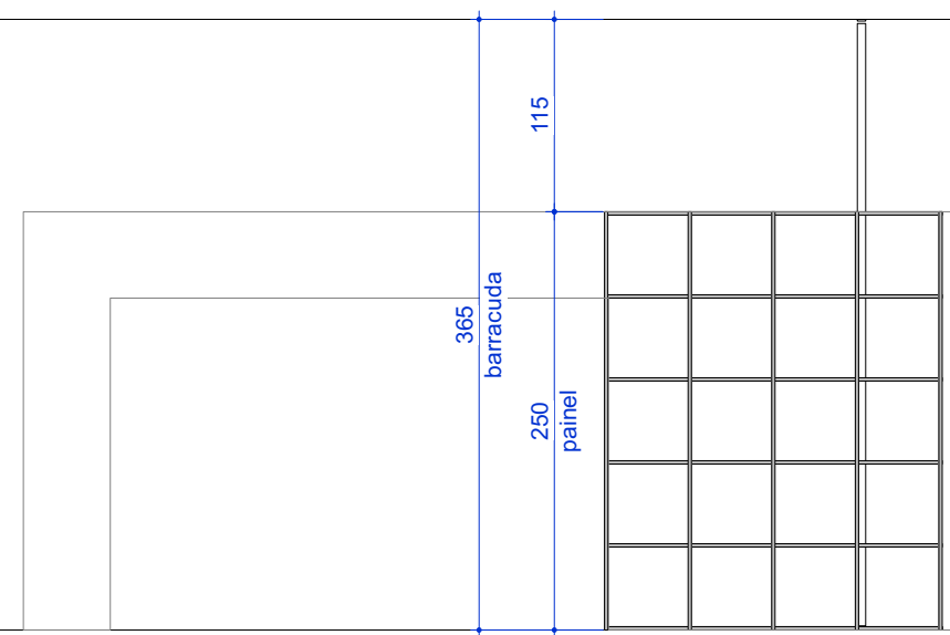
ELEVAÇÃO - PAINEL 1B1 escala 1:50
