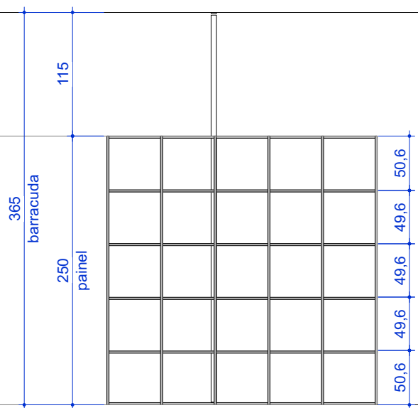
ELEVAÇÃO - PAINEL 1B2 escala 1:50
