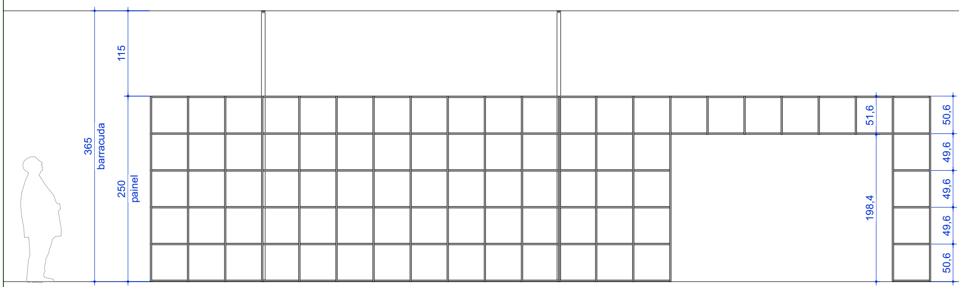
ELEVAÇÃO - PAINEL 1A escala 1:50
