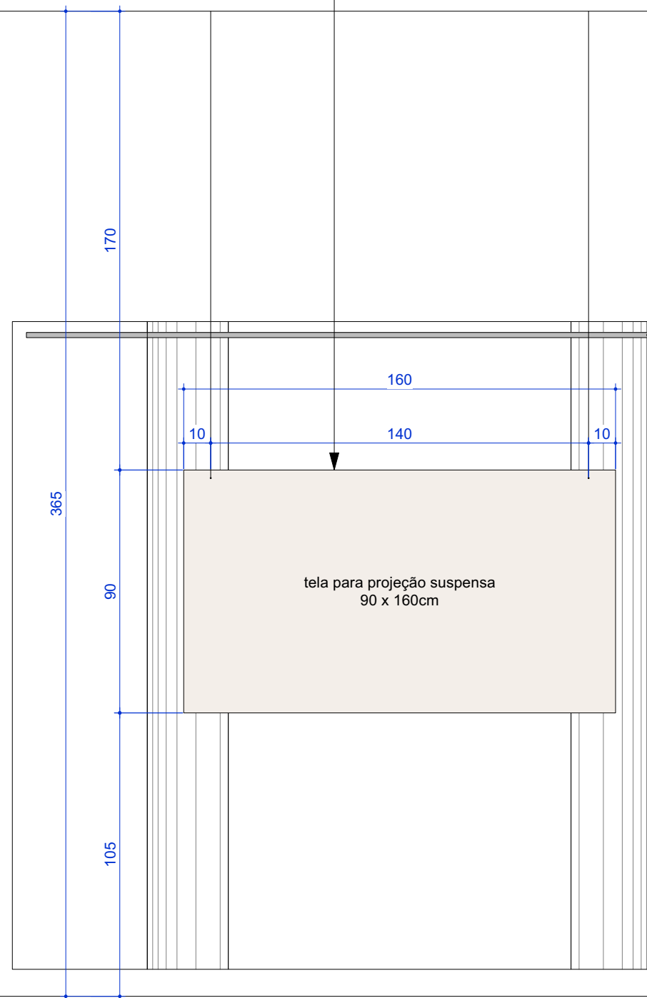
ELEVAÇÃO FRENTE - TELA PARA PROJEÇÃO escala 1:20
