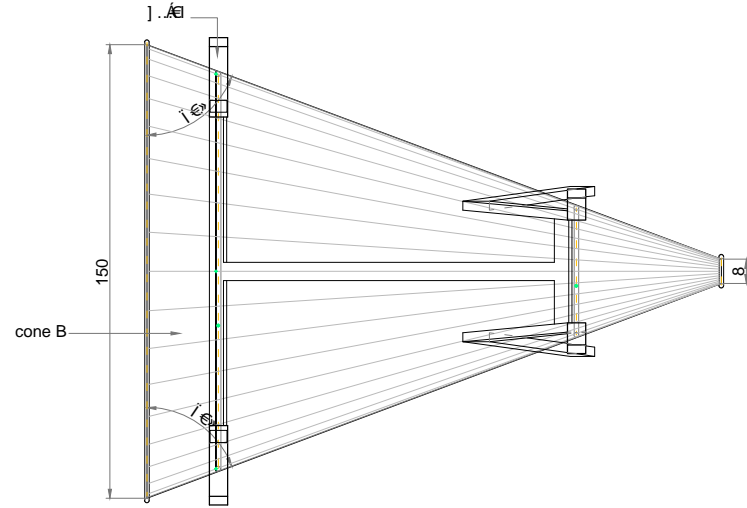
MODELO 04 - planta
