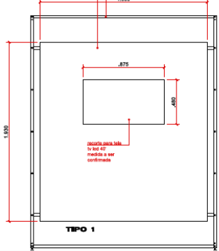
estrutura existente painel tipo 1 ref 20mm com acabamento de vinil adesivo frontal e pernas laterais no verso
