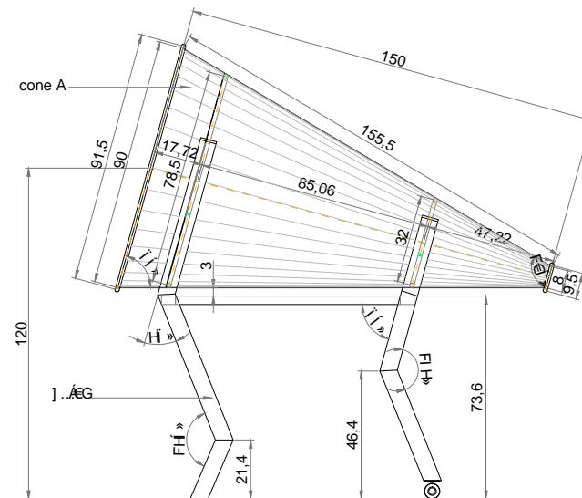
MODELO 02 - vista lateral
