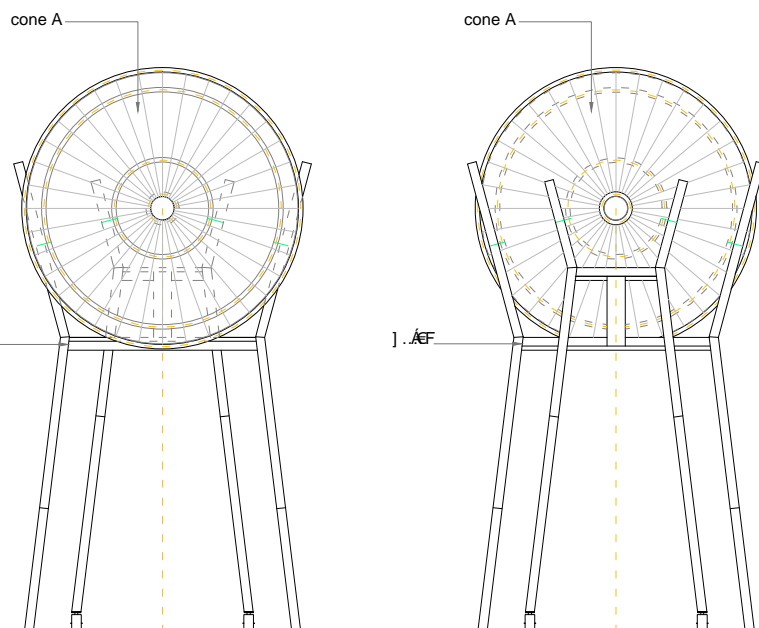
MODELO 01 - vista frontal
