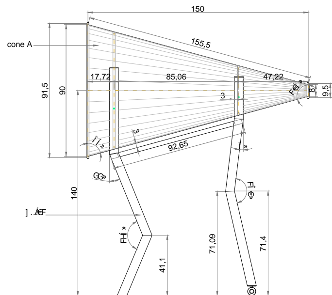
MODELO 01 - vista lateral
