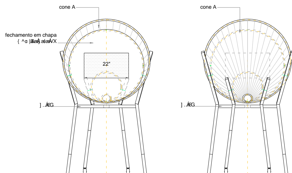
MODELO 02 - vista frontal
