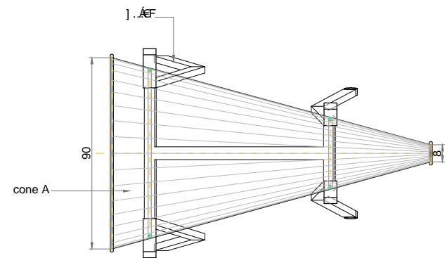
MODELO 01 - planta
