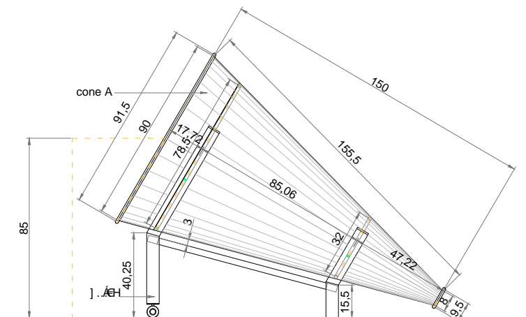
MODELO 03 - vista lateral
