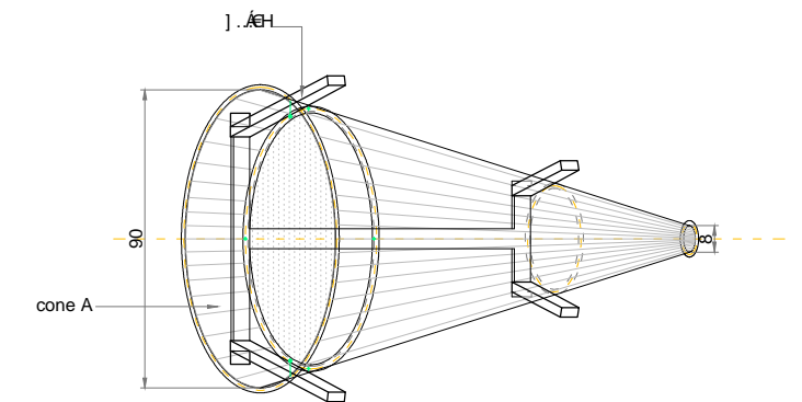
MODELO 03 - planta
