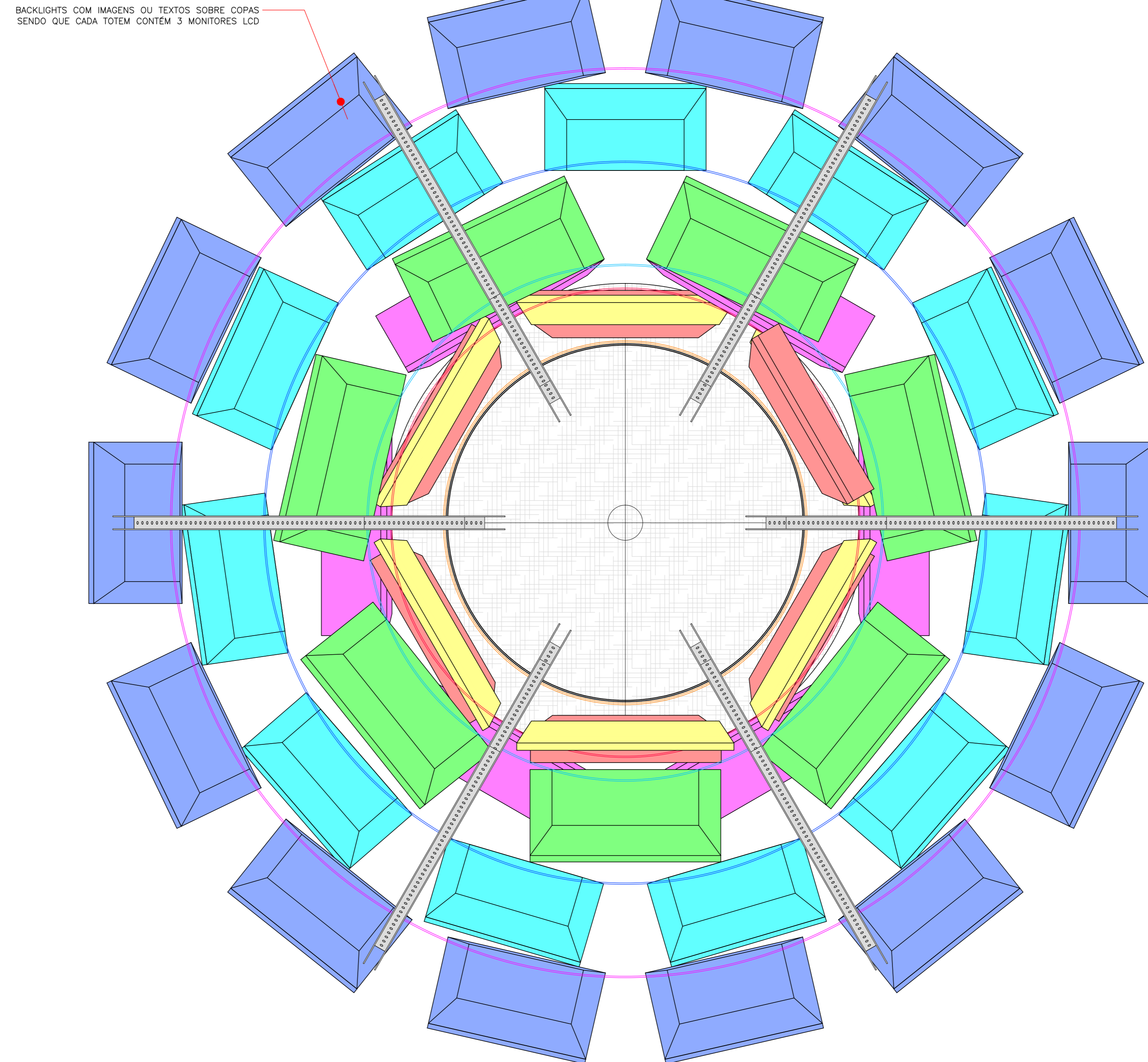
PLANTA COM BACKLIGHT E MONITORES ESC: 1:10
