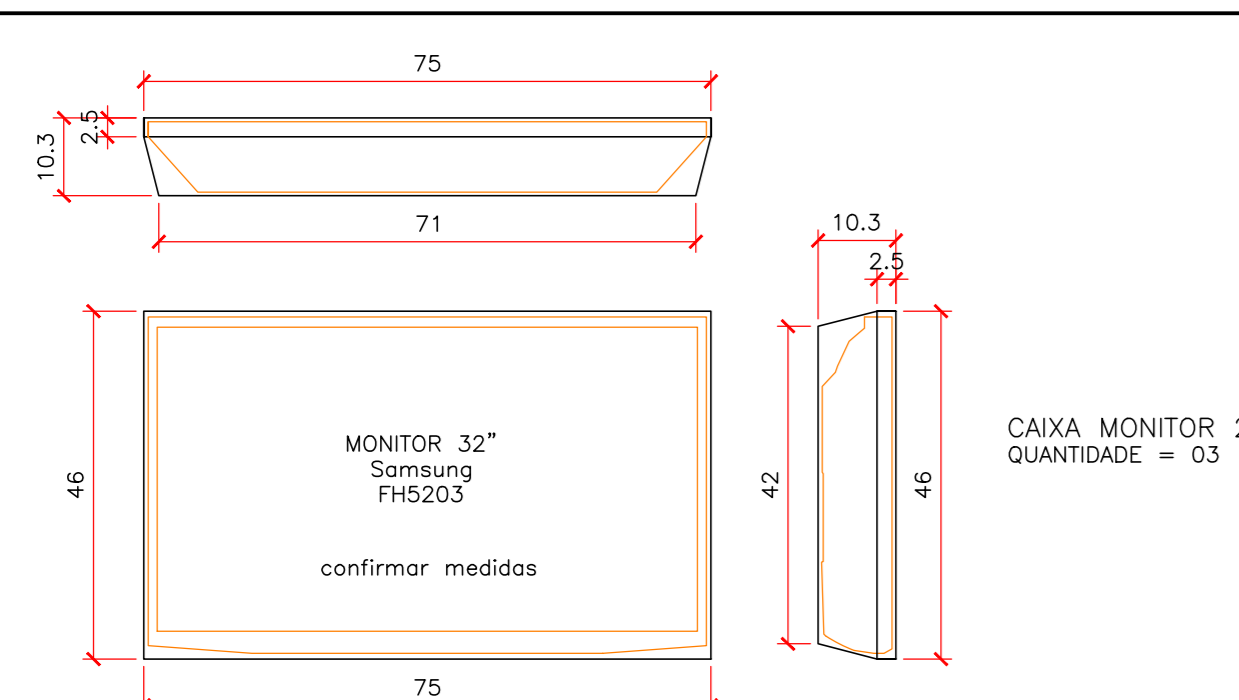
DETALHE COPAS-1 DIMENSÕES DOS BACKLIGHTS / ESC:1:10
